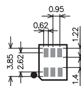
LT1790BIS6-2.5
