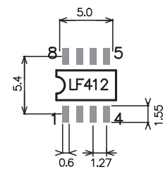
LF412CD
