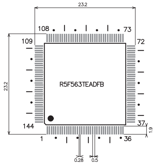
R5F563TEADFB
