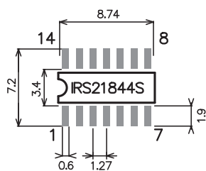
IRS21844S
